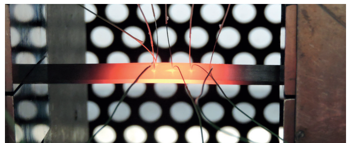
1 Versuch zur Nachstellung eines Wärmebehandlungsprozesses in der Prüfeinrichtung »Gleeble 3150«.
