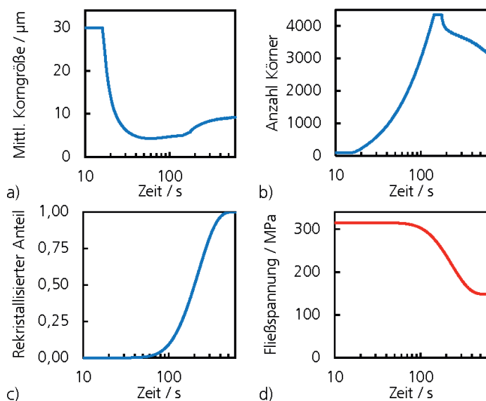
3 Rekristallisation nach dem Kaltwalzen (Dickenreduktion um 70 %): Entwicklung der Korngröße (a) und der Anzahl der Körner (b), rekristallisierter Anteil (c), Entwicklung der Fließspannung (d).
