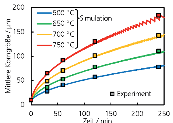
2 Simulation der Kornvergrößerung während der Wärmebehandlung von Kupfer und Vergleich mit experimentellen Ergebnissen (I. M. Ghauri et al.: J. Mater. Sci. 25, 1990).
